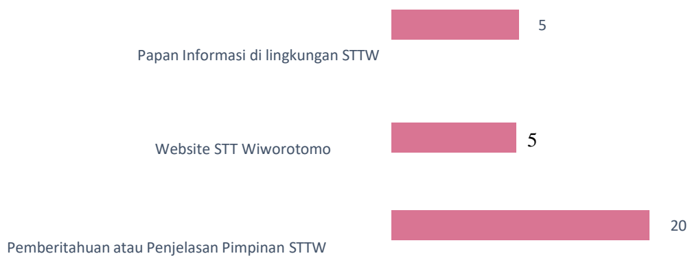
Gambar 3. 5 Grafik Pertanyaan 2
