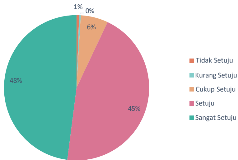
Gambar 3. 9 Grafik Pertanyaan 6
