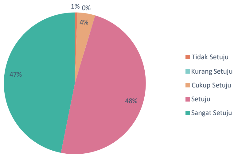
Gambar 3. 13 Grafik Pertanyaan 10
