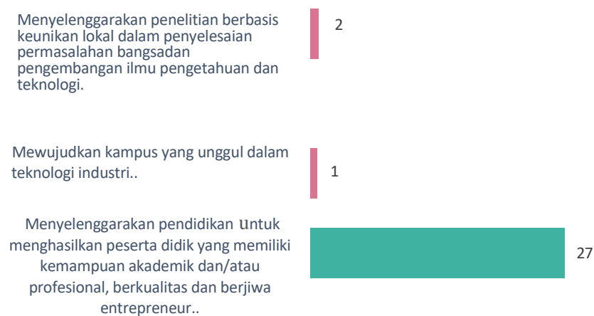
Gambar 3. 7 Grafik Pertanyaan 4
