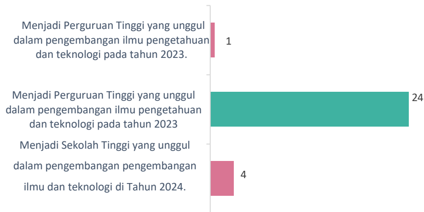
Gambar 3. 6 Grafik Pertanyaan 3
